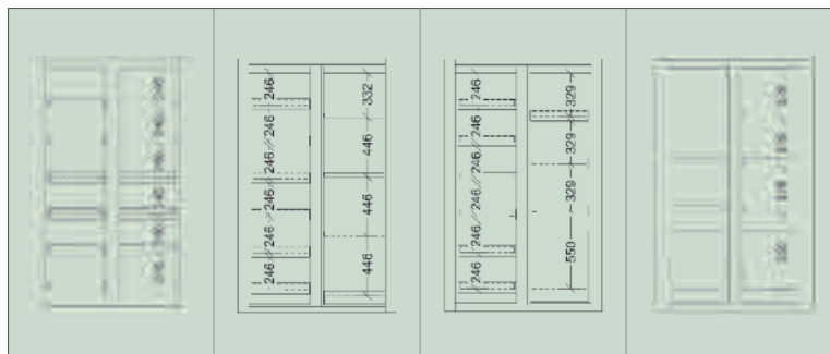
SIS Typ 90 / 1200 ES MI, Artikel-Nr. B80-2556-B, RAL 7035, inkl. 6 Auszugsböden (links) und 3 Auszugsböden sowie 1 Entsorgungsfach (rechts)
