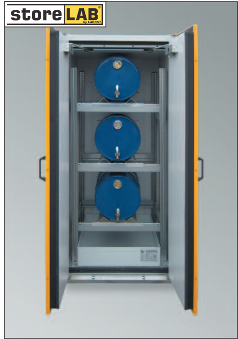
SiS-FAS Typ 90 / 900-360, Artikel-Nr. B80-2875-A
